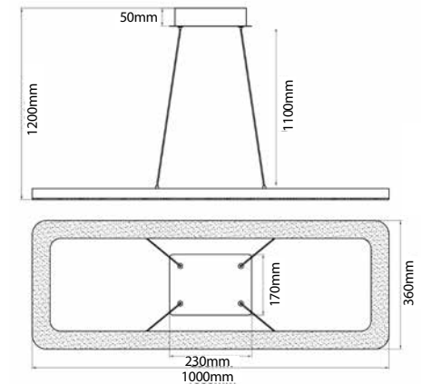
Crystal segment of the pendant
